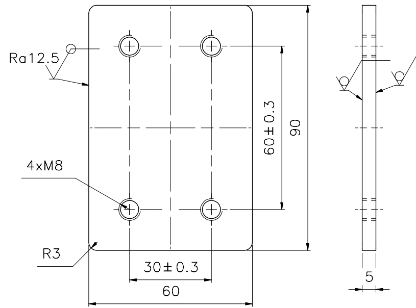
Item no.6 ( 1 : 1 )
